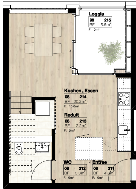
2.Obergeschoss
