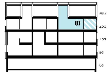
Längsschnitt
