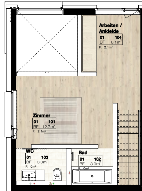
1. Obergeschoss
